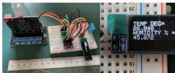
micro:bit の I2C インターフェイスにより 気温と湿度を計測して I2C ディスプレーに表示させた
